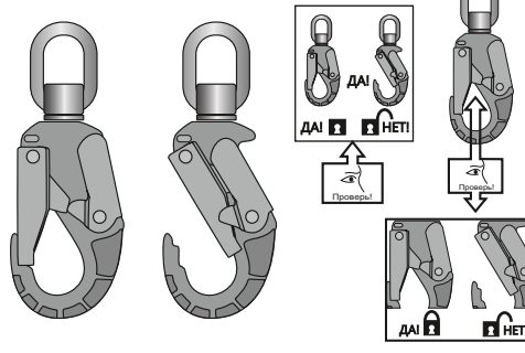
Рис. 6. Режимы работы устройства «НВ evak»
