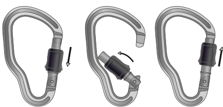
Рис. 3. Открытие / закрытие / фиксация запорного элемента
