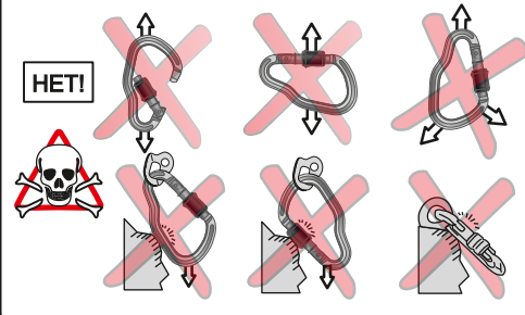
Рис. 5. Недопустимое использование
