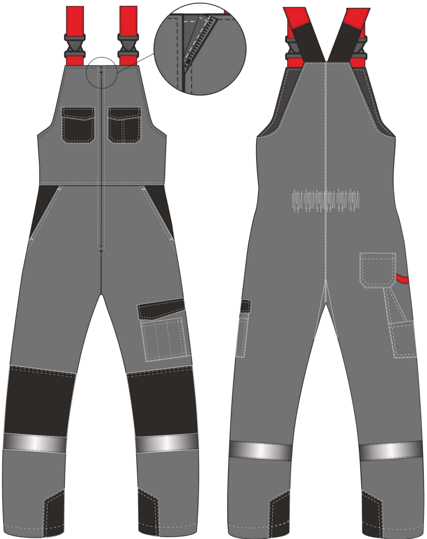
Рис. 4. Эскиз Костюм зимний Фаворит-Мега (тк.Протек,240) п/к, черный/красный/серый, Полукомбинезон, вид спереди и сзади.
