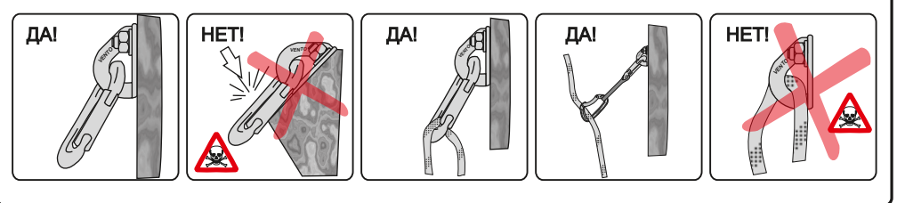
Рис. 7. Извлечение анкерного устройства
