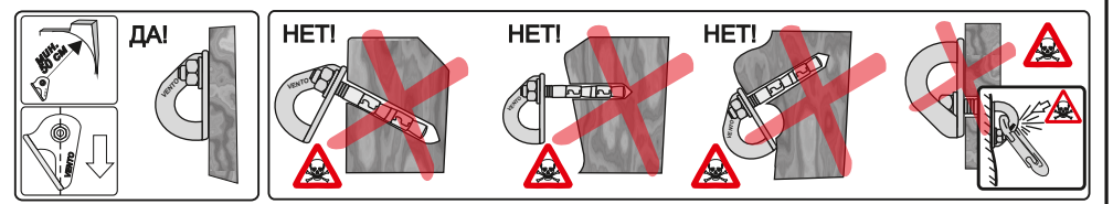
Рис. 5. Расположение анкерного устройства
