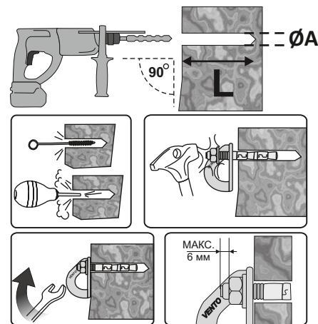
Рис. 4. Установка анкерного устройства
